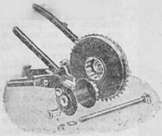
Фиг. 2. Современные конструкции. Выемная ось заднего колеса, при которой колесо удаляется, не трогая тормозной системы мотоцикла
